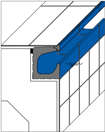
Details Beckenkopfsystem Bamberg, siehe Seite 30. For Details, pool edge system Bamberg, see page 30.
