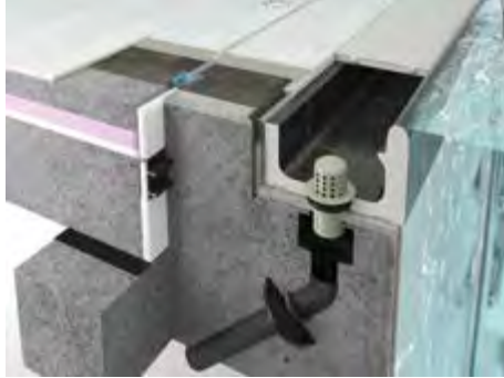
Großer Rinnenstein mit Handfasse, Abdeckrost und Flüsterablauf SILENT W 2000. Large gutter stone with handhold piece, cover grating and SILENT W 2000 outlet valve.
