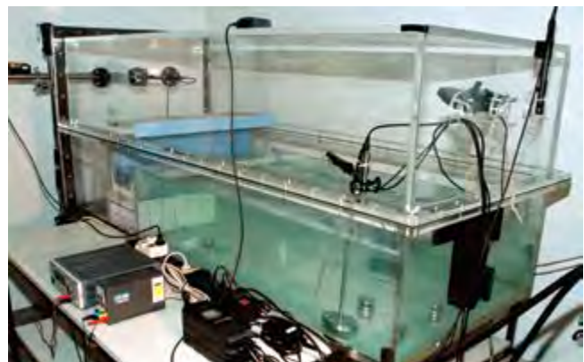
Wissenschaftliche Methoden und modernste Labortechnik liefern den Beweis zur Energieeffizienz der Bamberger Rinne. Scientific methods and state-of-the-art laboratory technology provide proof of the energy efficiency offered by the Bamberg Channel.
