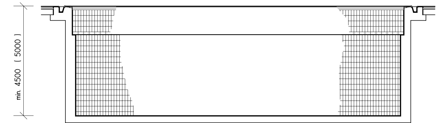
Schnitt/Coupe/Section/Sezione
