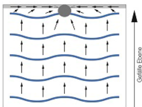
Prinzipdarstellung Kapillarwirkung
