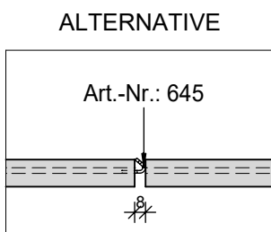
FUGENABSTANDSHALTER JOINT SPACER ENTRETOISE DE JOINTS
