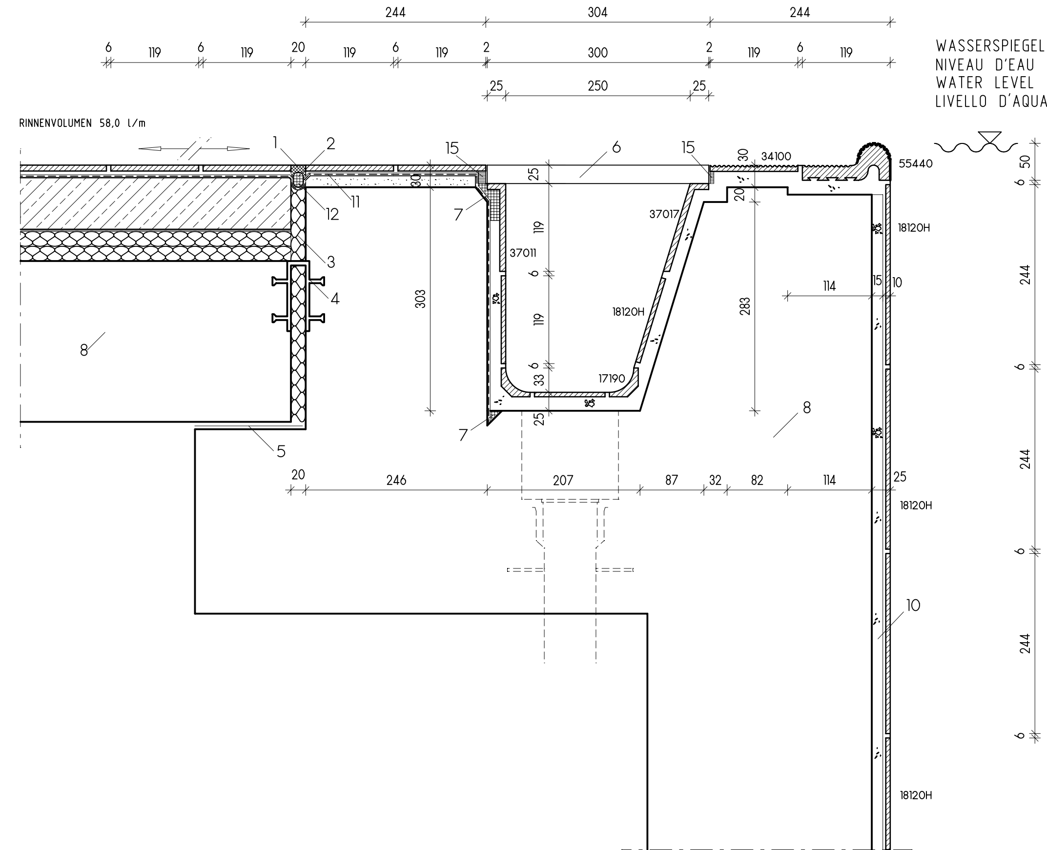
BECKENKOPFDETAIL M.:1:5
