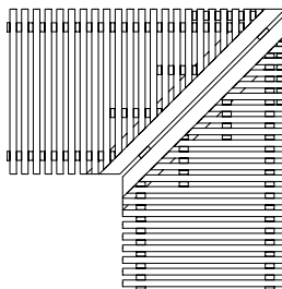
No. art. de esquina cortada a inglete: R21100 Emparrillado transversal de 250 mm de ancho
