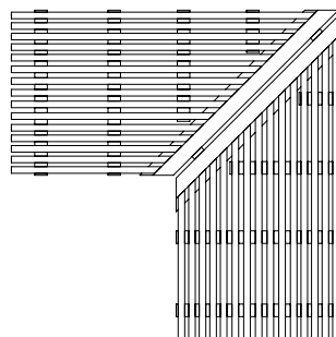
No. art. de esquina cortada a inglete: R51100 Emparrillado paralelo de 250 mm de ancho
