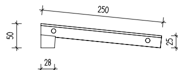
No. art.: R40100 Emparrillado transversal inclinado de 250 mm de ancho
