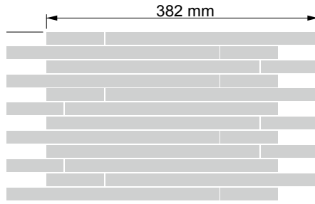
Bordüre Sola 24,3 x 43,8 cm, basalt, strukturiert
