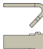
Artikel 645 Fugenabstandshalter K20/8 Gewicht: 0,5 kg/Karton Nennmaß: 4,8 x 10 mm Werkstoff: AlMg3 H22 (EN AW-5754) Kartoninhalt: 250 Stück schwarz beschichtet, RAL 7021
