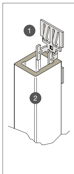
1 Befestigungsklammer
