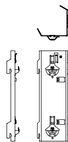
Artikel 705 OmegaV Außenecke blank* Werkstoff: AlMg3 H22 (EN AW-5754) unbeschichtet zur Montage von Gehrungsplatten und Außeneckprofilen
