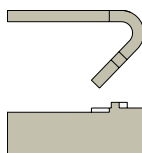
Artikel 645 Fugenabstandshalter K20/8 Gewicht: 0,5 kg/Karton Werkstoff: AlMg3 H22 (EN AW-5754) Kartoninhalt: 250 Stück schwarz beschichtet, RAL 7021
