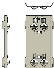
Art. 700 OmegaV con recubrimiento*, RAL 7021, Material: AlMg3 H22 (EN AW-5754) con recubrimiento negro para el montaje con junta distanciadora K20/8
