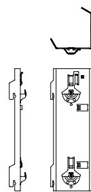
Art. 705 OmegaV ángulo saliente sin recubrimiento* Material: AlMg3 H22 (EN AW-5754) sin recubrimiento para el montaje de placas cortadas a inglete y perfiles para ángulos salientes
