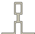
Art. 640Q Perfil para juntas Material: EN AW-6063 T66 con recubrimiento negro, RAL 7021
