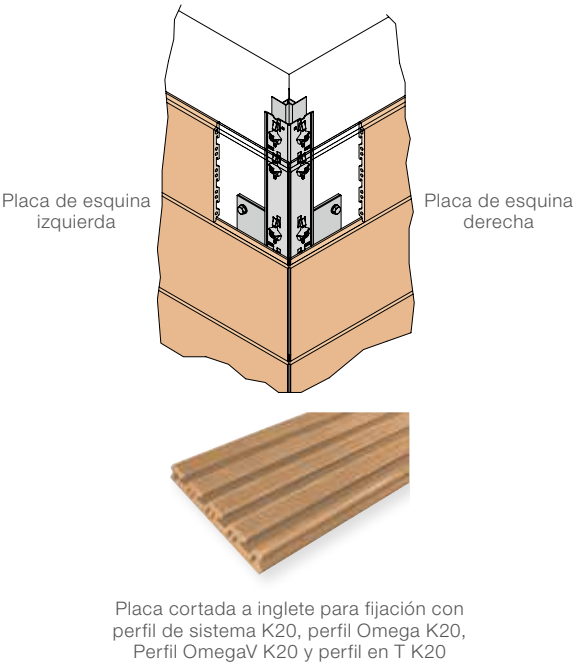
Solución para esquina con placa cortada a inglete y perfil de esquina exterior de espada
