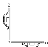
Art. 630 Perfil de sistema ángulo saliente* Material: AlMg3 H22 (EN AW-5754), sin recubrimiento para montaje de placas cortadas a inglete y perfiles de esquina exterior
