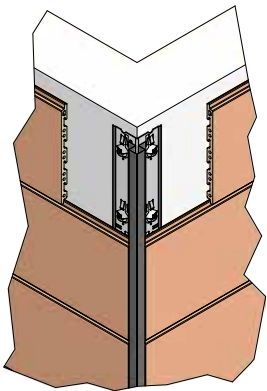
Solución de esquina con perfil de esquina exterior Cuadrado
