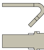
Art. 645 Junta distanciadora K20/8 Peso: 0,5 kg/caja Material: AlMg3 H22 (EN AW-5754) Contenido de la caja: 250 unidades con recubrimiento negro, RAL 7021
