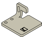
Art. 682R Garra en R Material: AlMg3 H22 (EN AW-5754), con recubrimiento negro
