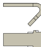
Art. 645 Junta distanciadora K20/8 Peso: 0,5 kg/caja Material: AlMg3 H22 (EN AW-5754) Contenido de la caja: 250 unidades con recubrimiento negro, RAL 7021
