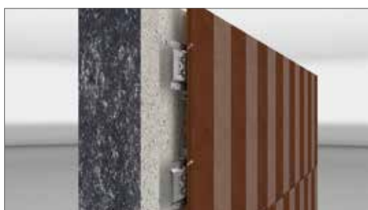
Bloqueo de las placas a los perfiles Omega K20 (con escuadra de bloqueo)
