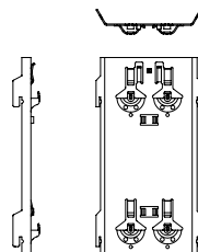
Art. 701 OmegaV sin recubrimiento* Material: AlMg3 H22 (EN AW-5754) sin recubrimiento para el montaje con perfil de junta OmegaV K20/8
