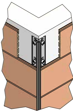
Solución de esquina con perfil de esquina exterior Negativo
