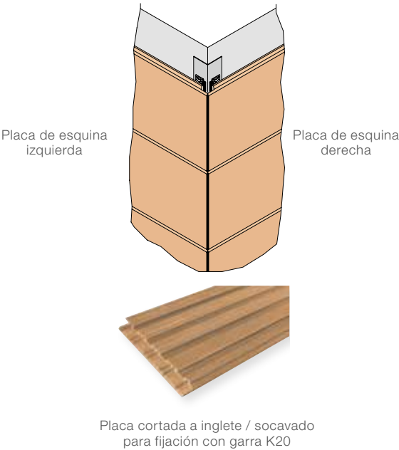
Solución para esquina con placas cortadas a inglete
