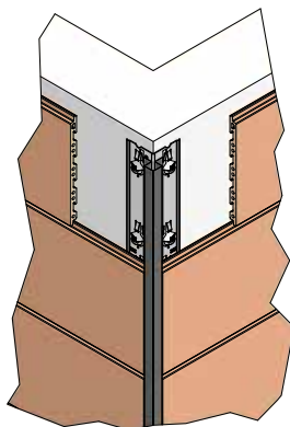
soluzione per angoli con profilato per angoli esterni, quadrato
