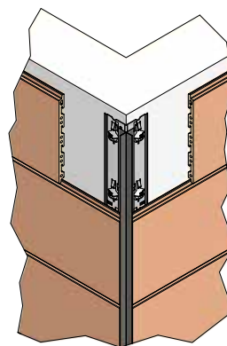
soluzione per angoli con profilato per angoli esterni, negativo
