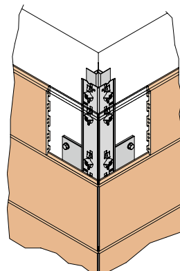
soluzione con lastra d'angolo e profilato per angoli esterni, sporgente
