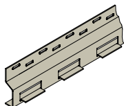
articolo 710 profilato di appoggio OmegaS verniciato materiale: AlMg3 H22 (EN AW-5754) verniciato in nero, RAL 7021
