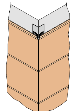
soluzione con lastre d'angolo
