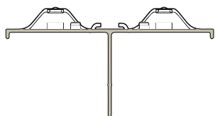
articolo 695Q profilato a T K20* materiale: EN AW-6060 T6 anodizzato C35, RAL 7021, per montaggio con profilato per giunti 640Q e distanziatore K20/8
