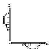
articolo 630 profilato per sistemi, angolo esterno* materiale: AlMg3 H22 (EN AW-5754), non verniciato per montaggio di lastre d'angolo e profilati per angoli esterni
